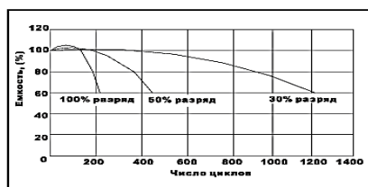
График зависимости ёмкости от количества циклов
