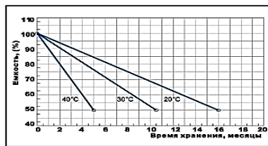
График зависимости ёмкости от времени хранения
