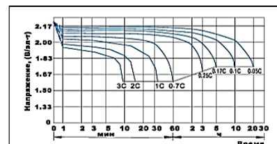
Разрядные кривые постоянным током
