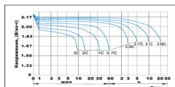
Разрядные кривые постоянным током
