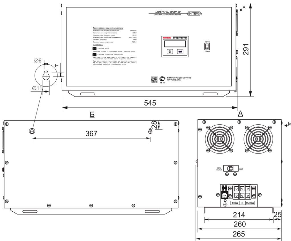
Габаритные и установочные размеры стабилизаторов напряжения переменного тока LIDER PS1200W-30
