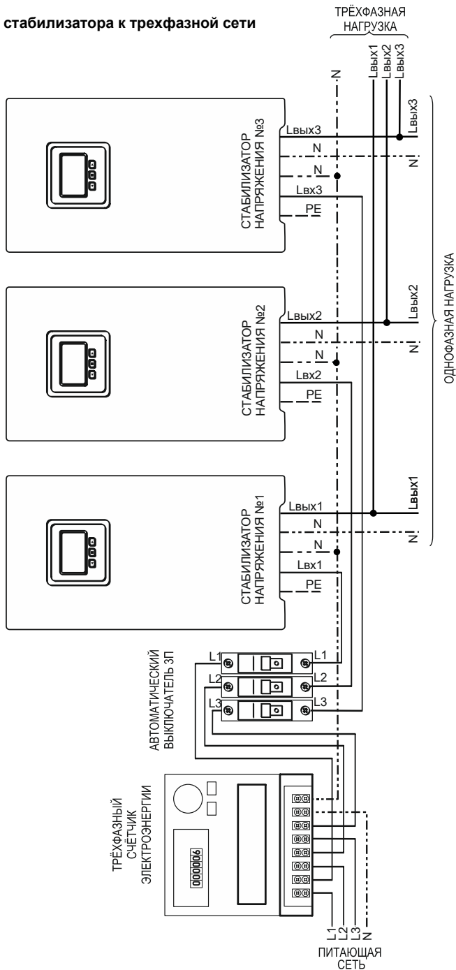
Рисунок 5 - Схема подключения стабилизатора к трехфазной сети.
