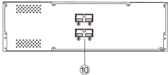
Monolith B 6000RT(LT)/10000RT(LT) и батарейный блок
