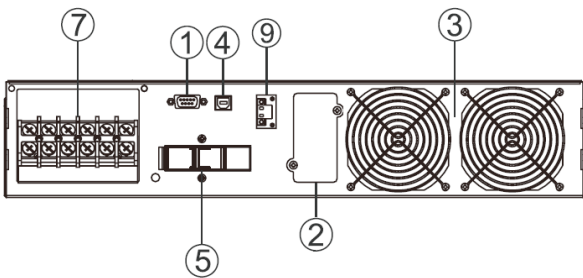
Monolith B 6000RT(LT)/10000RT(LT) и батарейный блок
