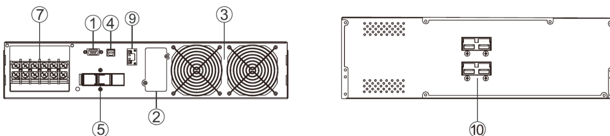
Monolith B 6000RT(LT)/10000RT(LT) и батарейный блок
