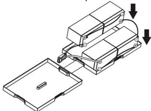
Рисунок 10. Порядок сборки комплекта из четырех батарей.
