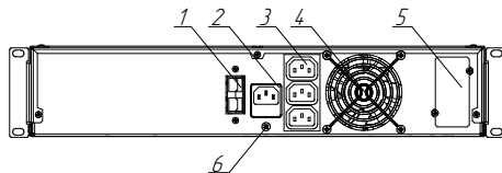
Рисунок 5б. Компоненты задней панели ИБП Штиль STR500SL-18
