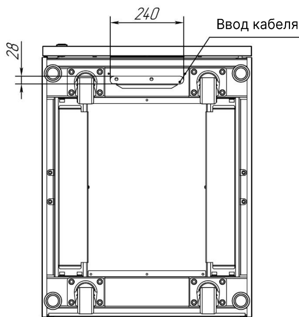
Вид снизу
